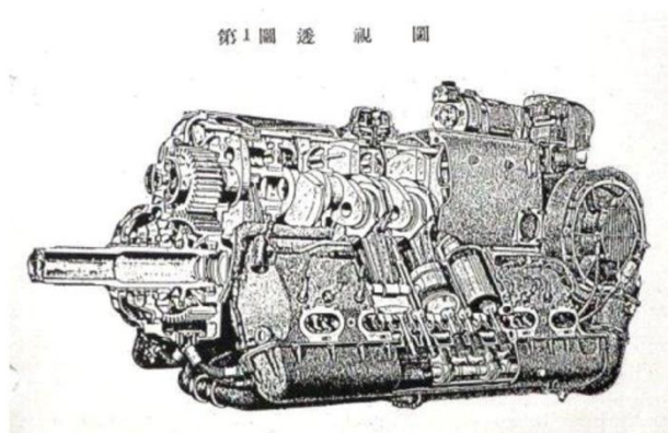
①アツタ発動機 30型 透視図
