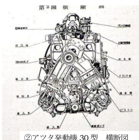
②アツタ発動機 30型 横断図
