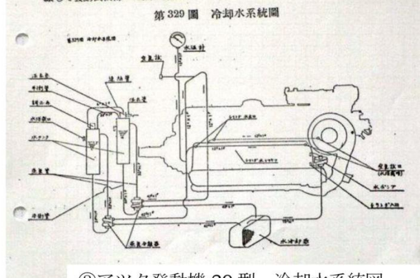
③アツタ発動機 30型 冷却水系統図
